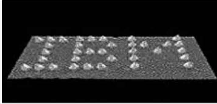
Şekil 3.7: 35 Ksenon Atomuyla Hecelenmiş Olan IBM Logosu, 1989
